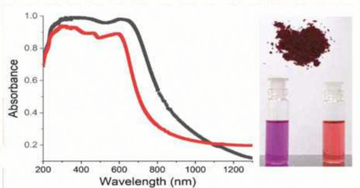
कार्बनिक पॉलिमर का ओवरलैड यूवी-विज़-एनआईआर स्पेक्ट्रा
